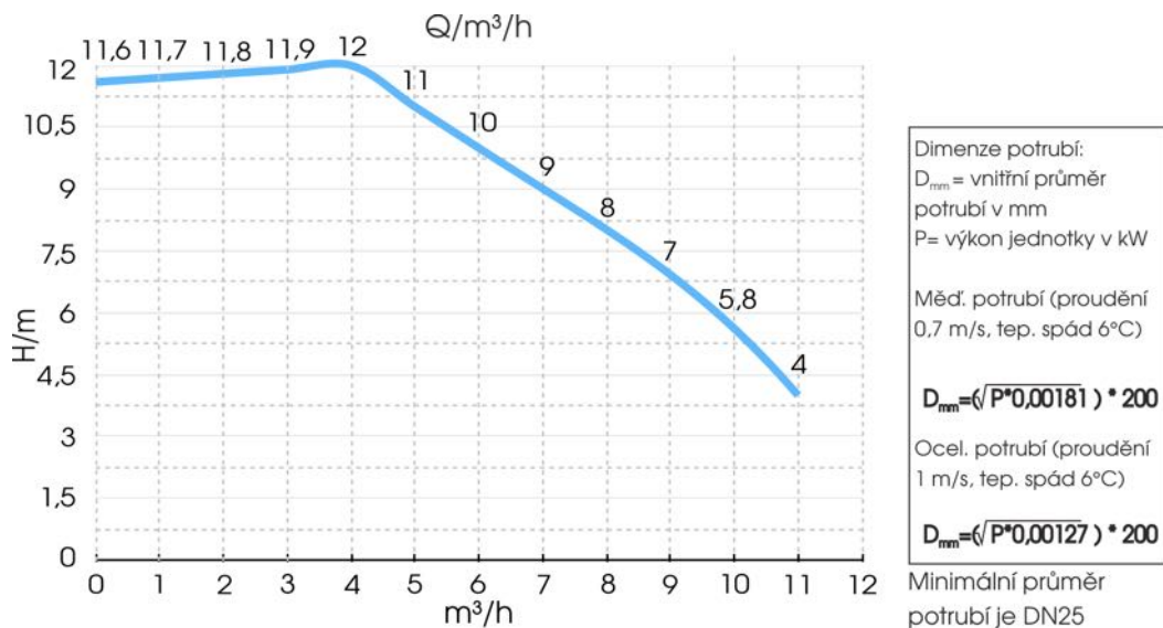
Obrázek 8.1: Parametry hydraulického výkonu vnitřní jednotky (včetně kompletního vybavení)
