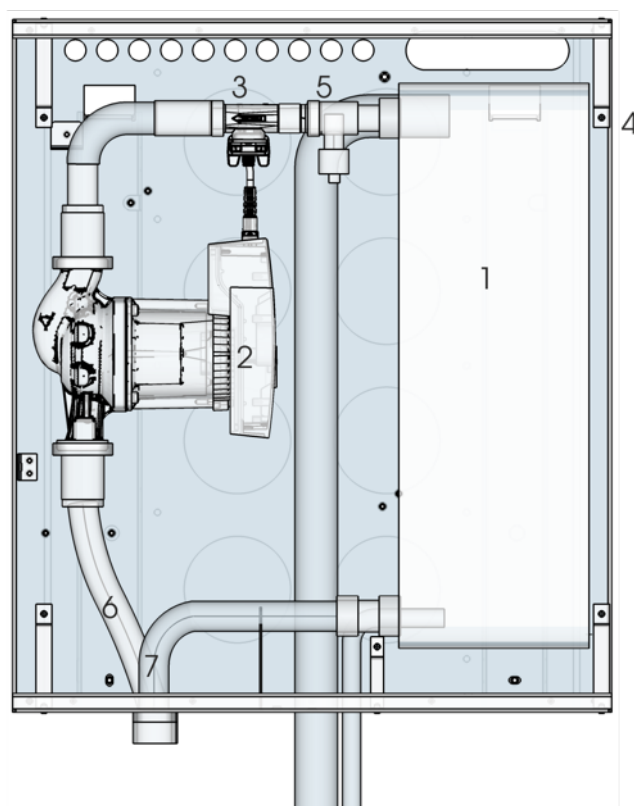
Obrázek 9.2: Schéma hydraulického zapojení vnitřní jednotky
