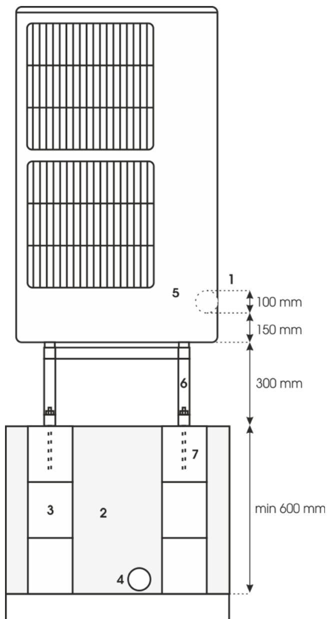
Obrázek 3.2: Náčrtek základu pro venkovní jednotku - čelní pohled 1 - prostup skrz stěnu domu do vnitřního prostoru; 2 - drenážní jáma; 3 - betonová tvárnice; 4 - drenážní hadice; 5 - venkovní jednotka; 6 - konzole s antikorozií; 7 - svorník pro uchycení konzoly
