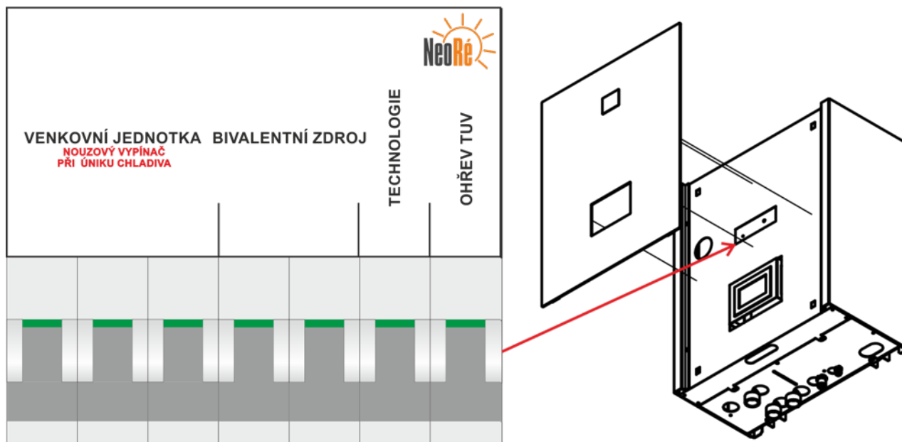
Obrázek 4.1: Jistící prvky tepelného čerpadla
