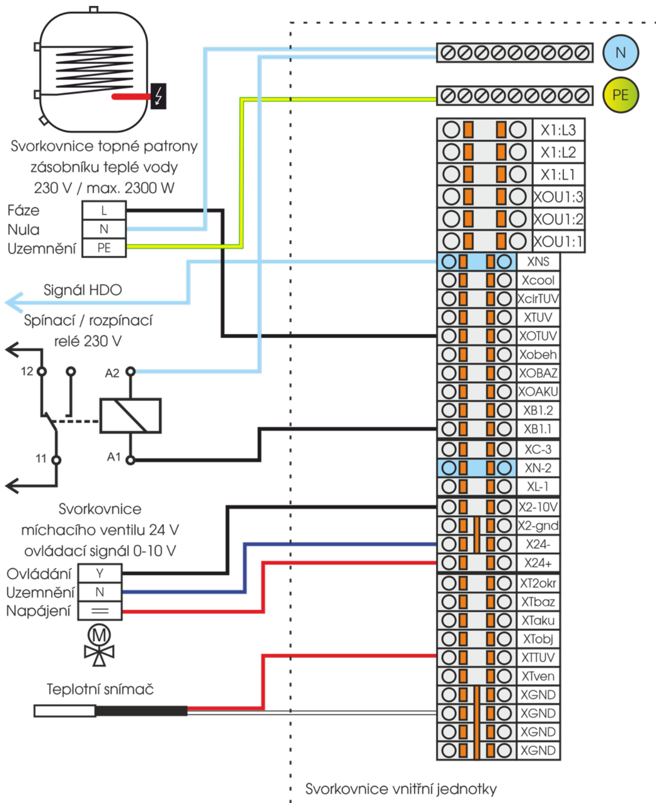
Obrázek 3.10: Svorkovnice vnitřní jednotky a ovládaných zařízení
