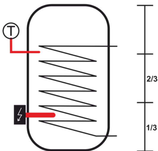
Obrázek 3.11: Dimenzování zásobníku teplé vody
