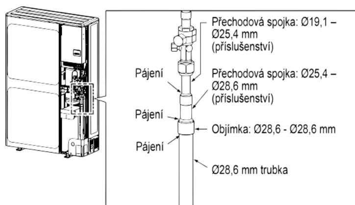
Obrázek 3.6: Přechodová spojka na straně plynu - adaptér z 19,1 mm na výslednou 28,6 mm
