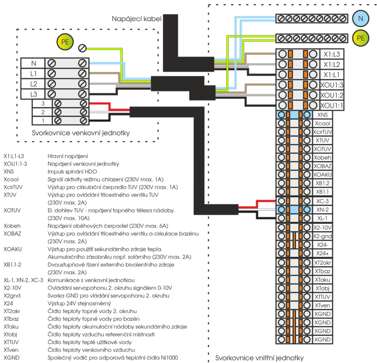
Obrázek 3.9: Svorkovnice vnitřní a venkovní jednotky a jejich propojení
