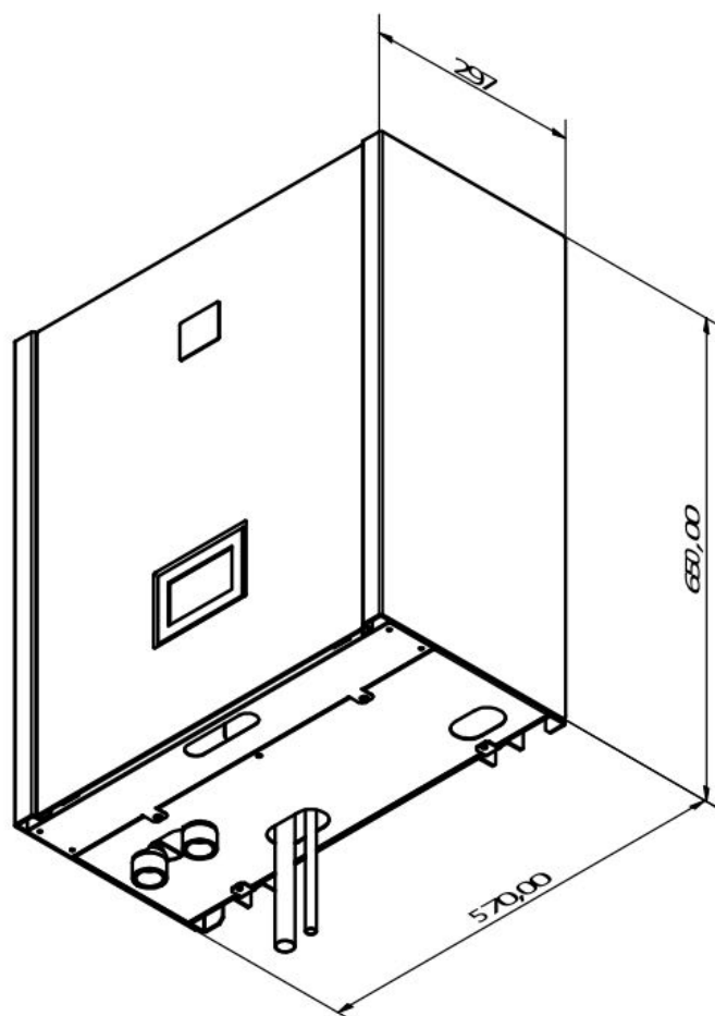
Obrázek 9.4: Rozměry
