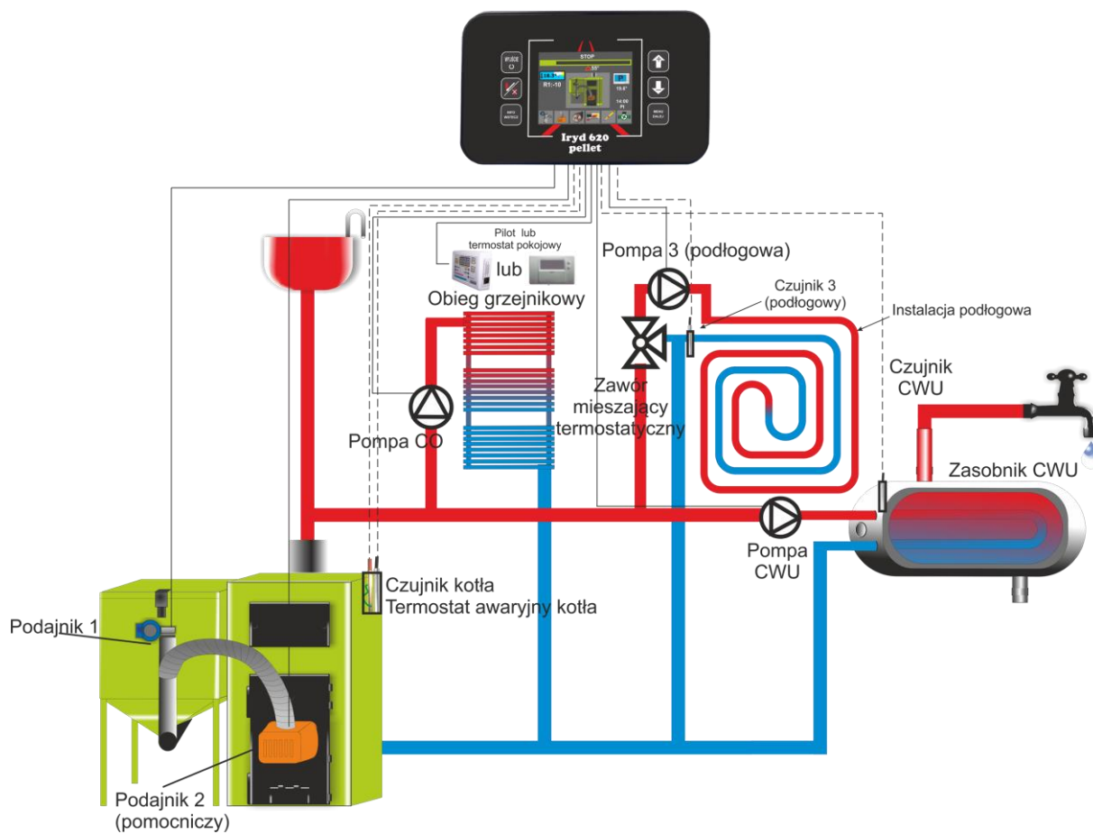
Instalacje s čerpadlem 3 – Podlahové topení
