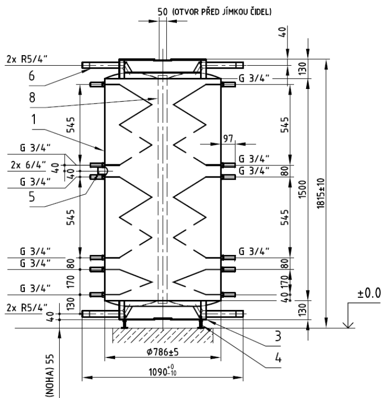
POHLED "Q" - NÁDOBA PAST 750
