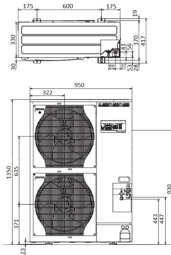
PUHZ-SHW80VAA / YAA
