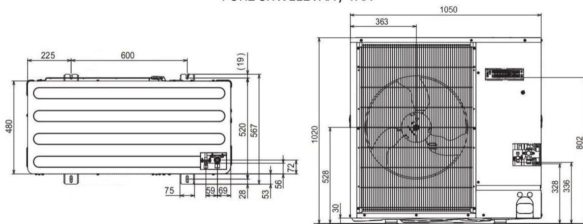
PUHZ-SHW112VAA / YAA
