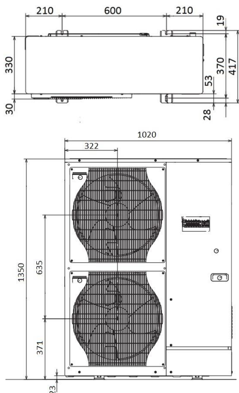
PUHZ-SHW80VAA / YAA
