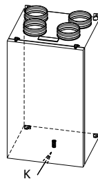
DUPLEX ECV5 – ze spodní strany
