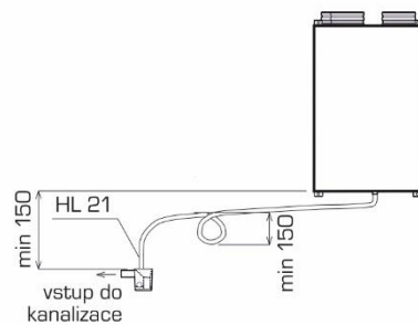
DUPLEX ECV5 – svislé provedení
