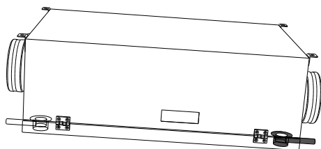
DUPLEX EC5 – podstropní provedení Na nižší straně (výfuk i 2 ) napojit Na vyšší straně (e 2 ) zaslepit zátkou
