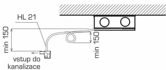
DUPLEX EC5 – podstropní provedení
