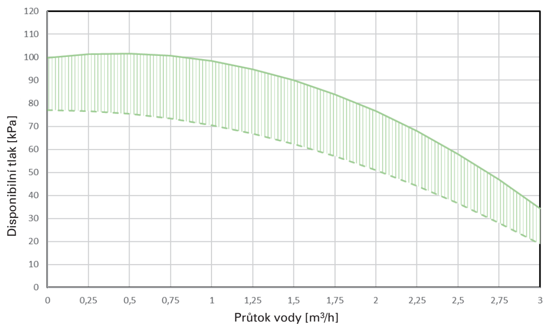
14, 16, 18 Pracovní oblast oběhového čerpadla
