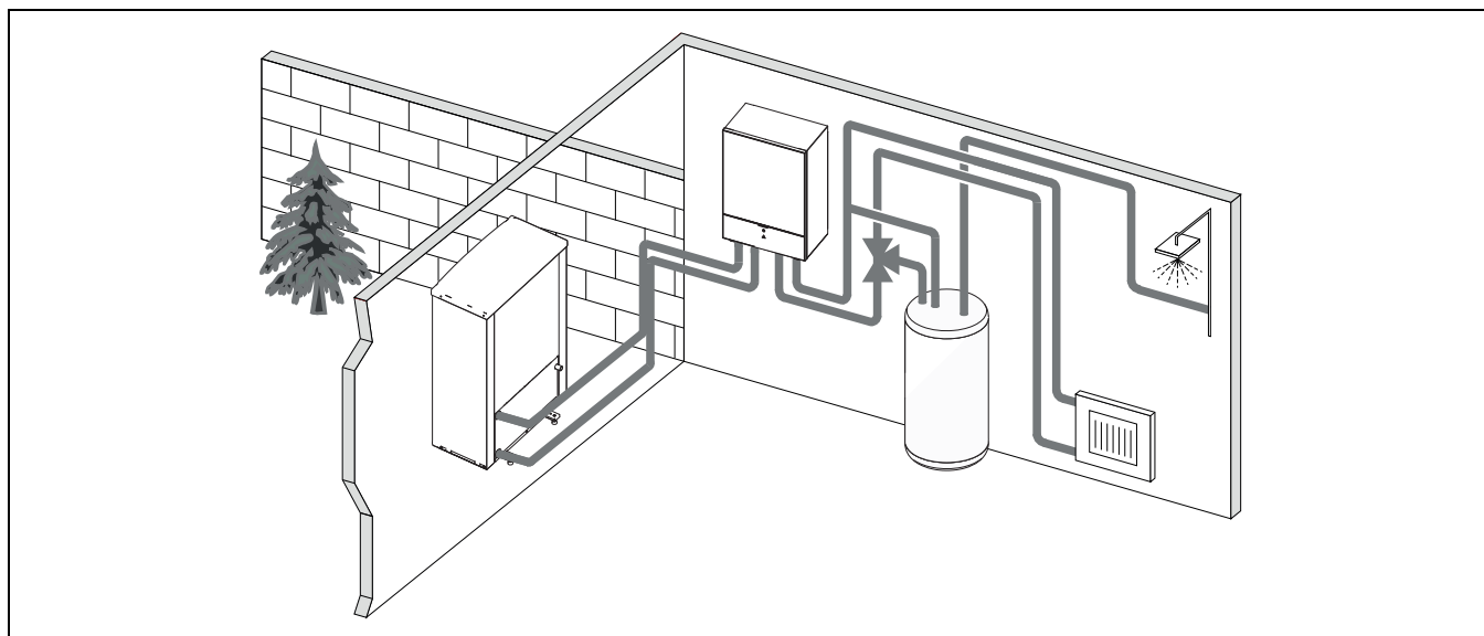
Obr. 3 Tepelné čerpadlo Compress 7000i AW, vnitřní jednotka AWE s elektrickou pomocnou topnou tyčí a externím zásobníkem teplé vody
