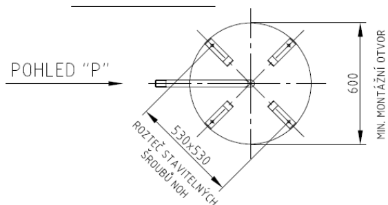
PŮDORYS PAST
