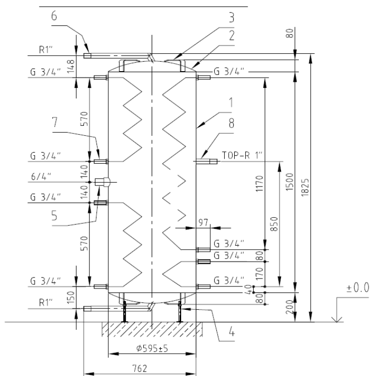
POHLED "Q" - NÁDOBA PAST 425
