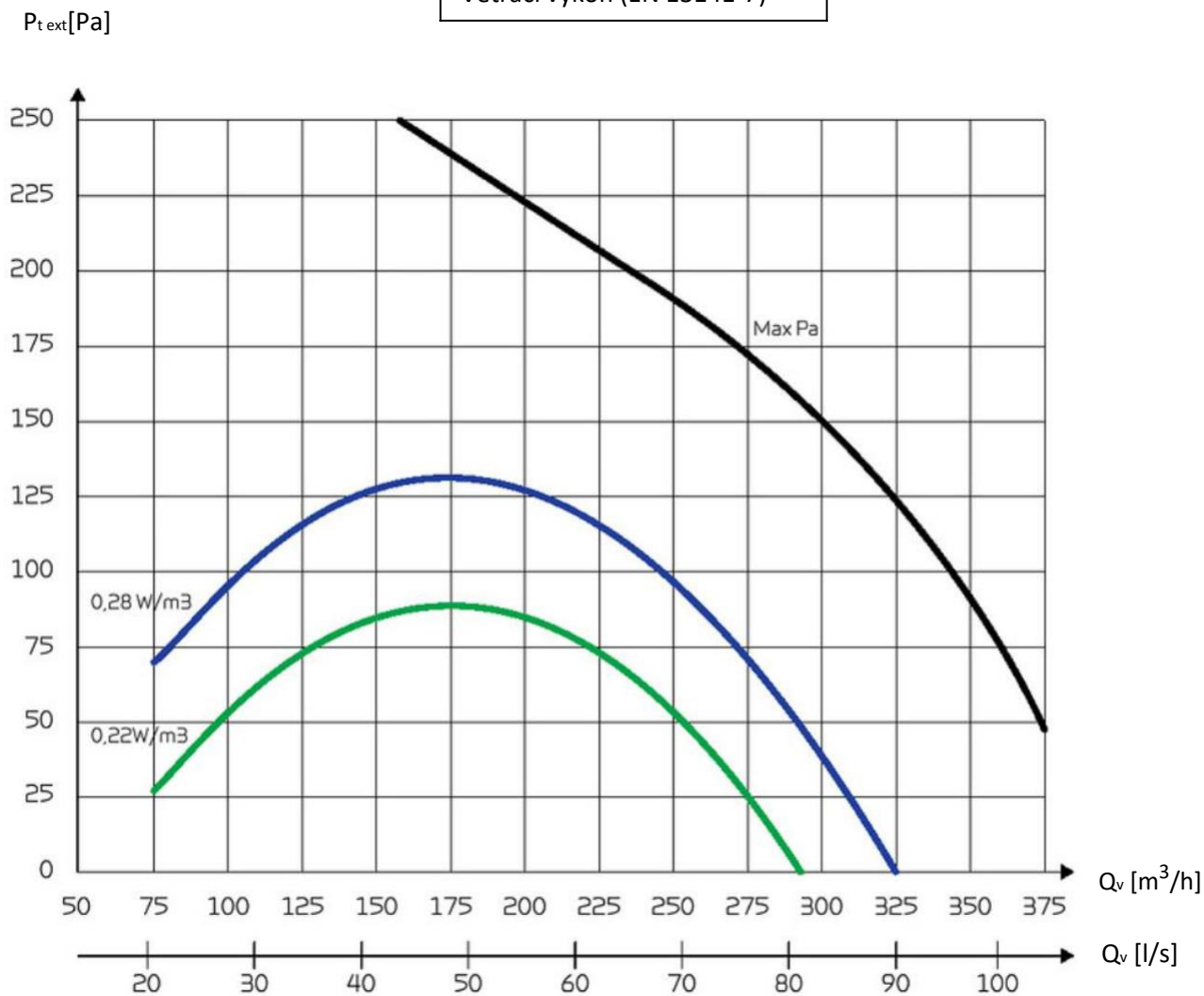
Větrací výkon (EN 13141-7)
