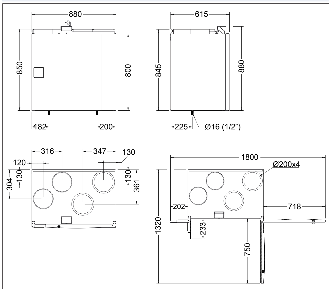
Obr. 1 Levý model (přívod čerstvého vzduchu je umístěn na levé straně)
