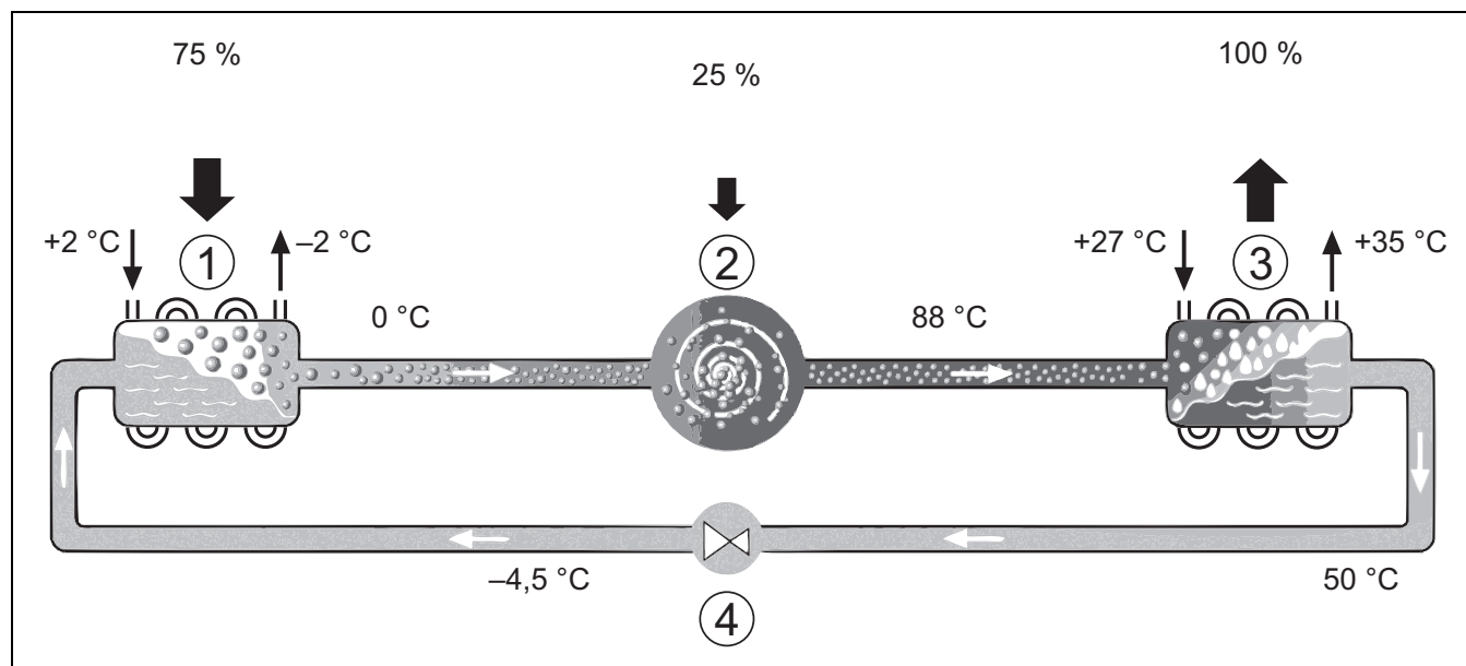
Obr. 6 Princip funkce okruhu chladiva v tepelném čerpadle
