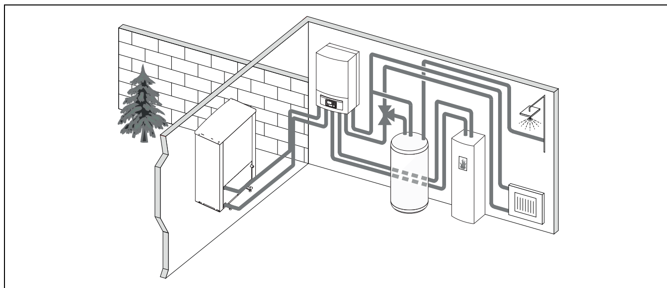
Obr. 3 Tepelné čerpadlo WPL AR, vnitřní jednotka IDU B bez elektrické pomocné topné tyče, externí zásobník teplé vody a externí dohřev
