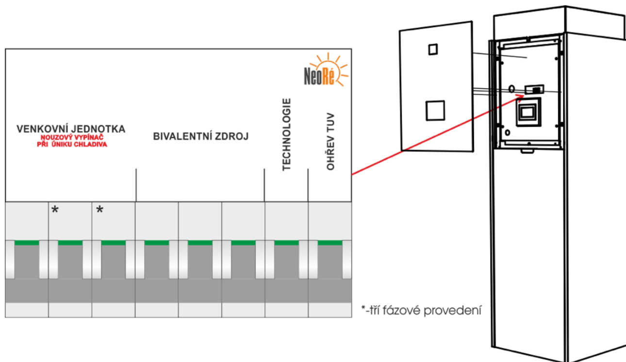
Obrázek 5.1: Jistící prvky tepelného čerpadla
