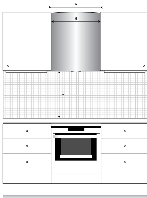
Obr. 3 SAVE VTR 150/K v kuchyňské lince
