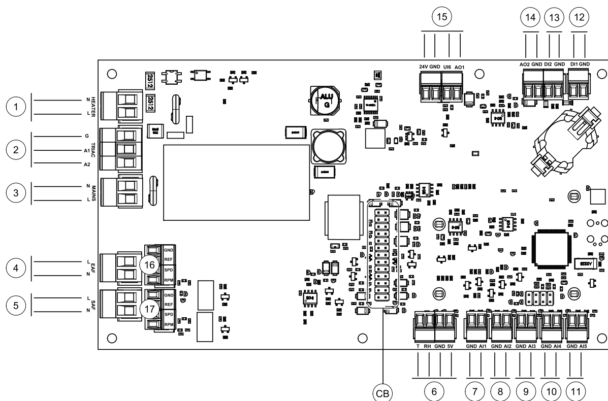
Obr. 5 Připojení hlavní řídicí desky
