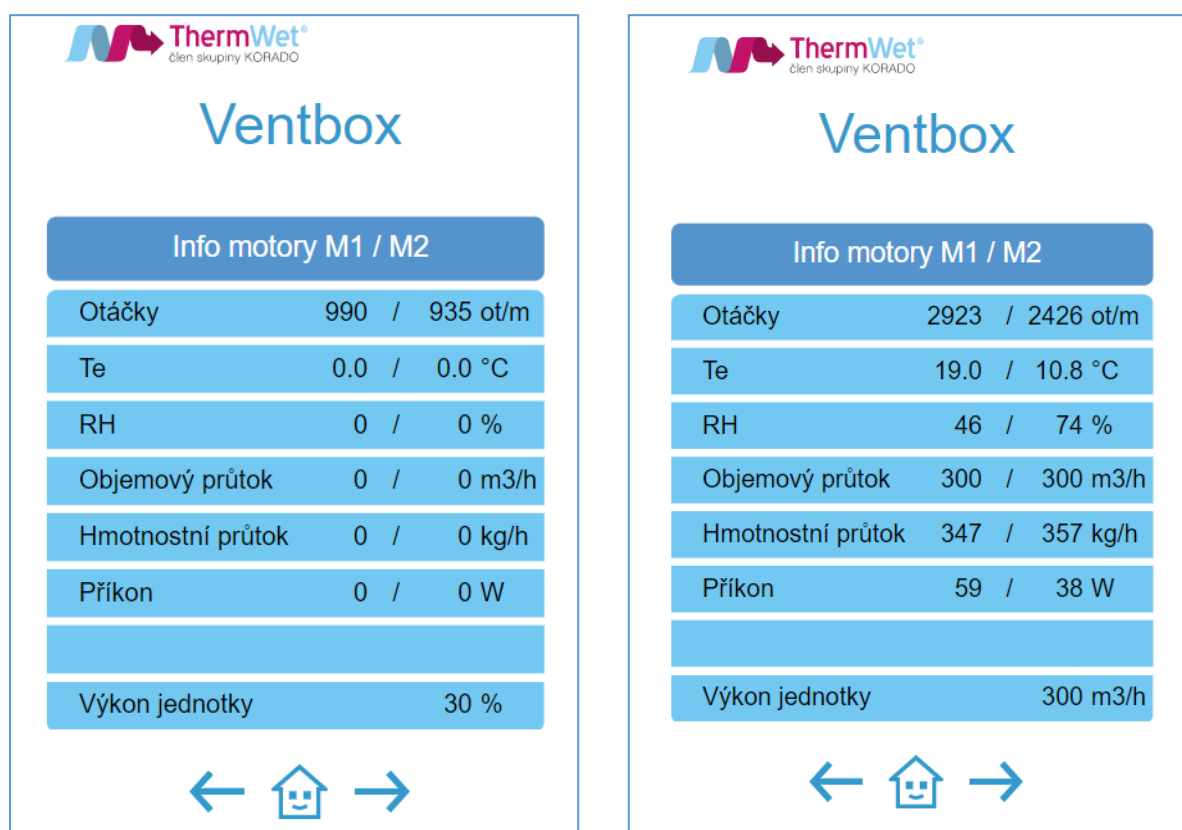
Obrázek 23: Aktuální hodnoty čidel ventilátorů OPTIMUM / PREMIUM
