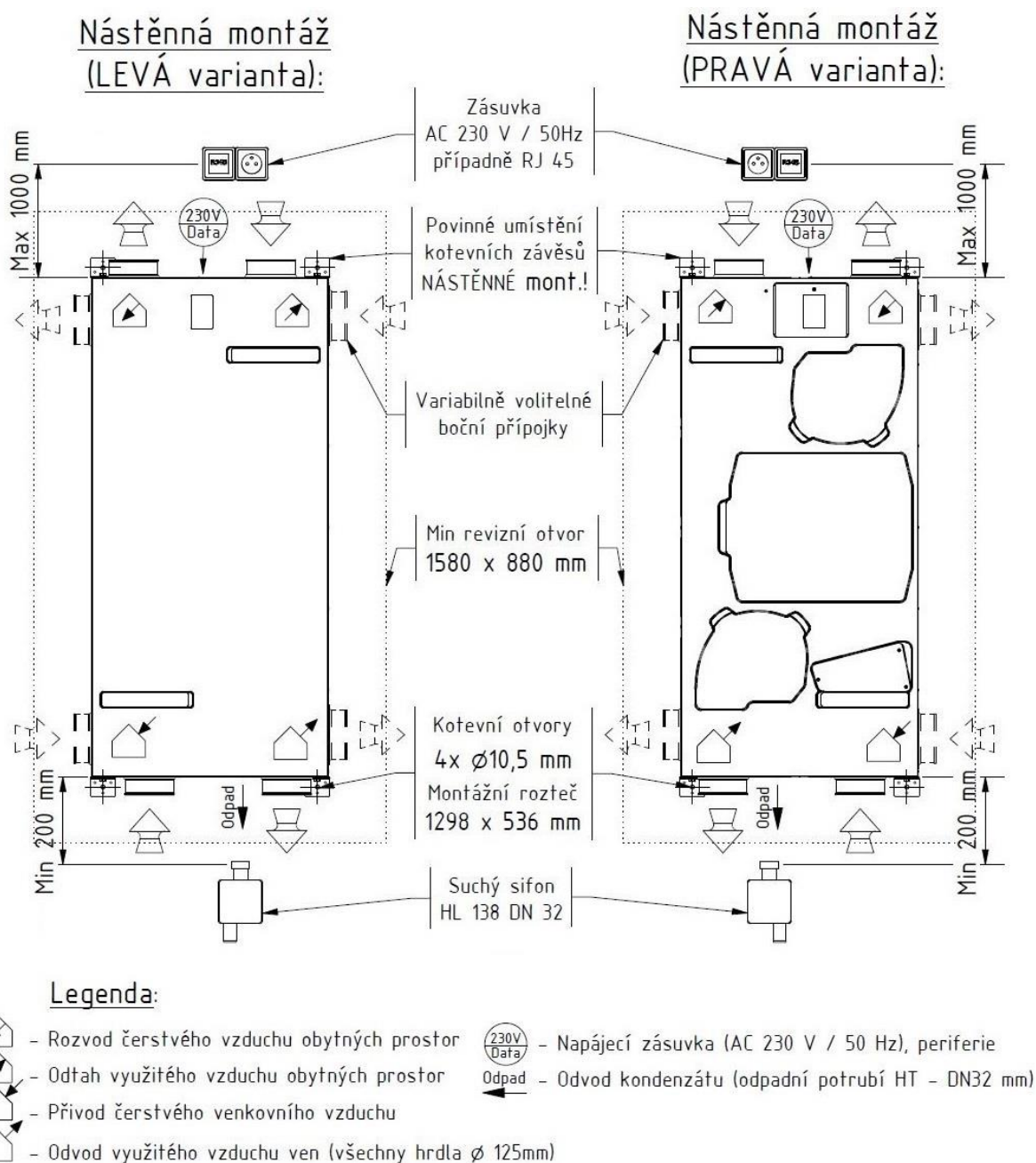
Obrázek 32: Instalační prostor pro „Nástěnnou montáž“
