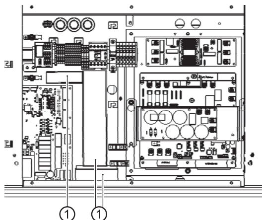
1 Kabelový kanál
