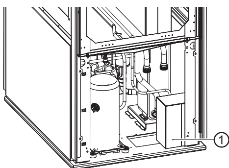
Kompaktní jednotka s hermeticky uzavřeným kompresorem, všemi bezpečnostně důležitými prvky pro monitorování chladicího okruhu a hadicí pro odvod kondenzátu (připojená na straně tepelného čerpadla).
