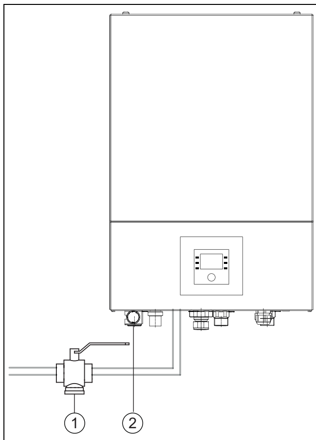
Obr. 6 Inneenhet AWE
