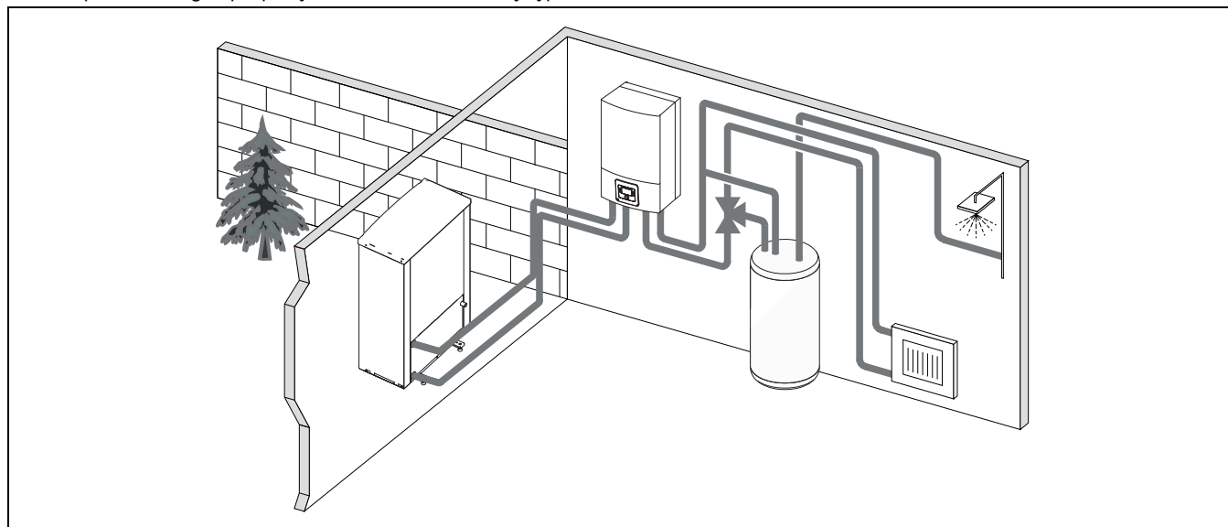
Obr. 3 Tepelné čerpadlo Compress 7000 AW, vnitřní jednotka AWE s elektrickou pomocnou topnou tyčí a externím zásobníkem teplé vody
