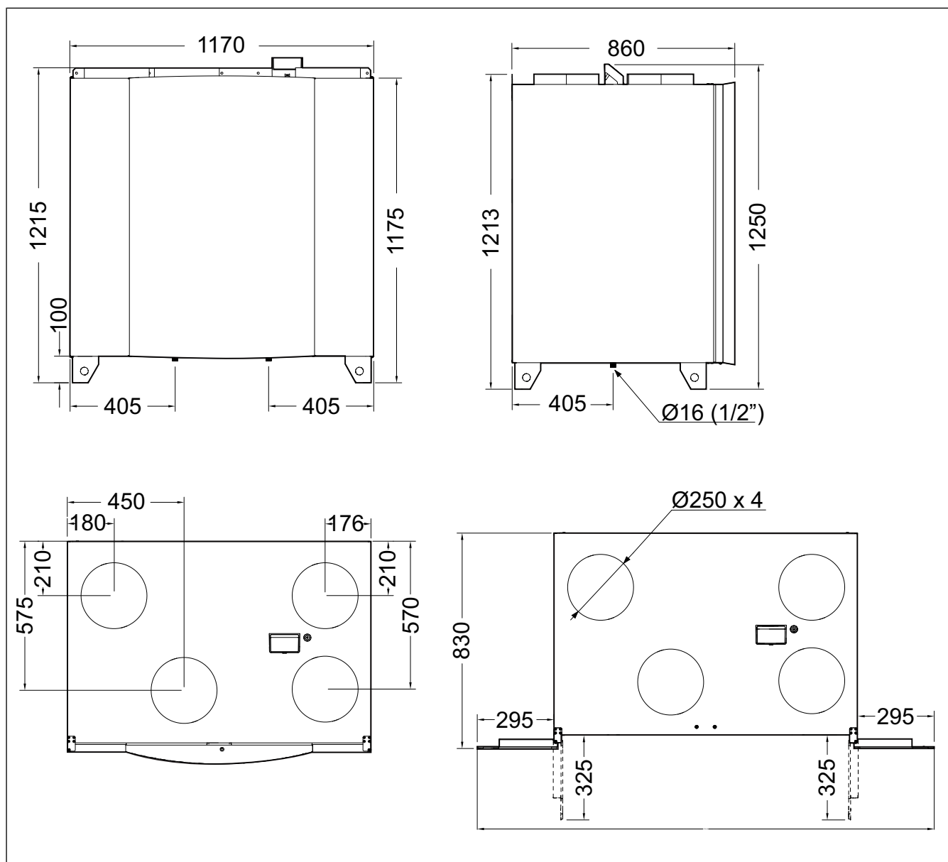
Obr. 2 Pravý model (přívod čerstvého vzduchu je umístěn na pravé straně)
