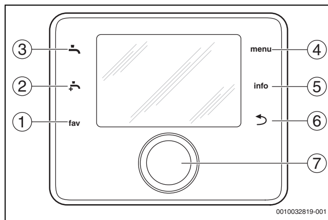
Obr. 4 Ovládací prvky
