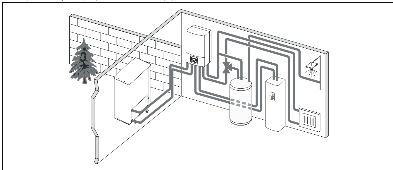
Obr. 3 Tepelné čerpadlo Compress 6000 AW, vnitřní jednotka AWB bez elektrické pomocné topné tyče, externí zásobník teplé vody a externí dohřev
