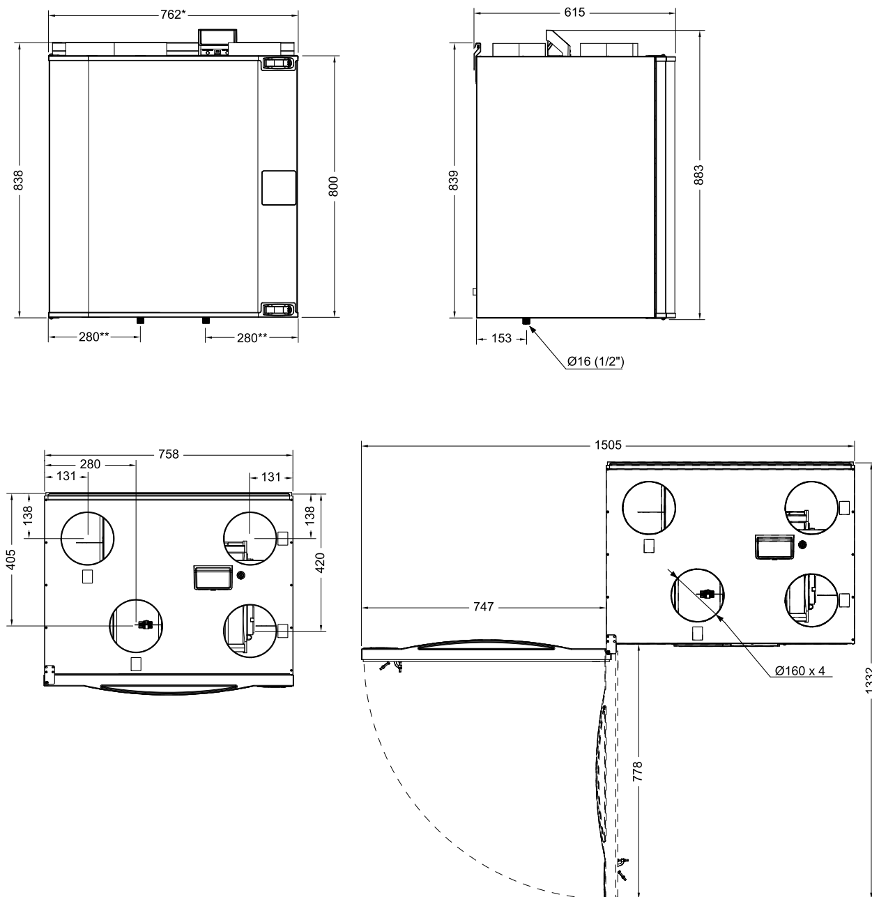
Obr. 2 Rozměry pravého modelu
