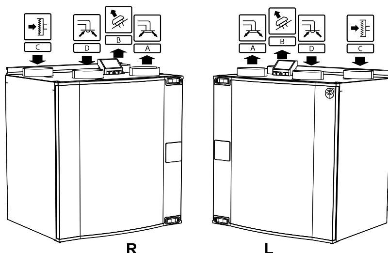
Obr. 3 Připojení potrubí
