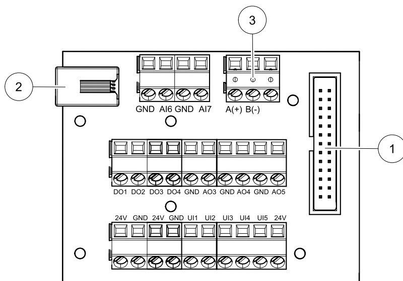
Obr. 6 Externí svorkovnice
