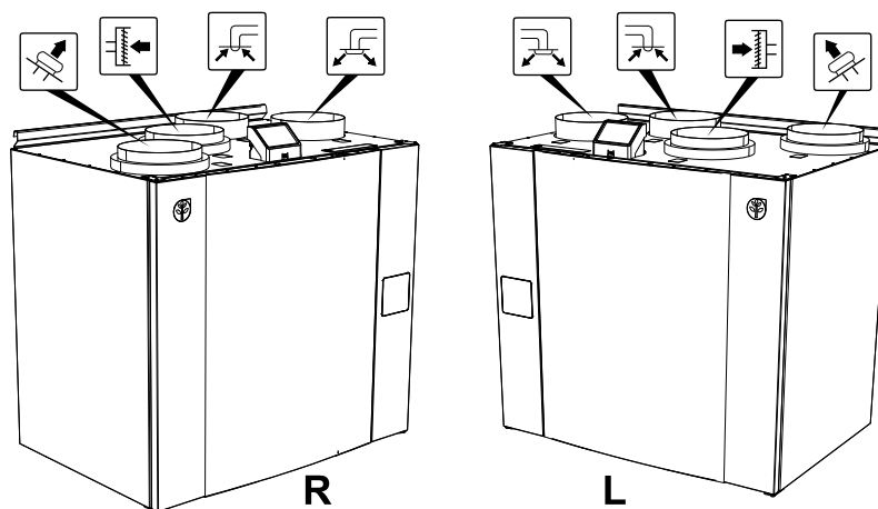
Obr. 4 Připojení potrubí
