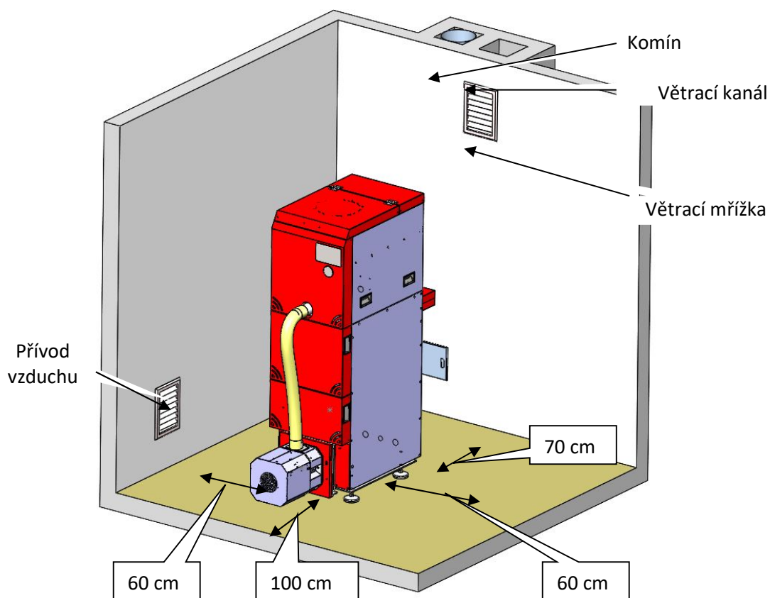
Obrázek 5. Ukázková kotelna s přívodní a odvodní ventilací, komínem a minimálními servisními vzdálenostmi od stěn a přepážek.
