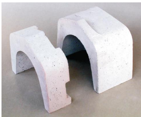
Obr. č. 7 Keramický reflektor - dvojdielný
