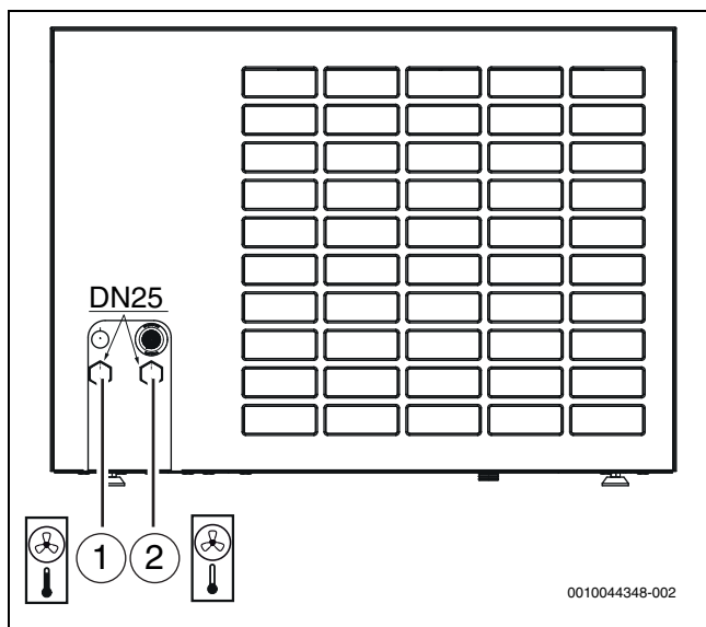
Obr. 29 Potrubní připojení teplotnosné látky, popis se vztahuje na všechny velikosti
