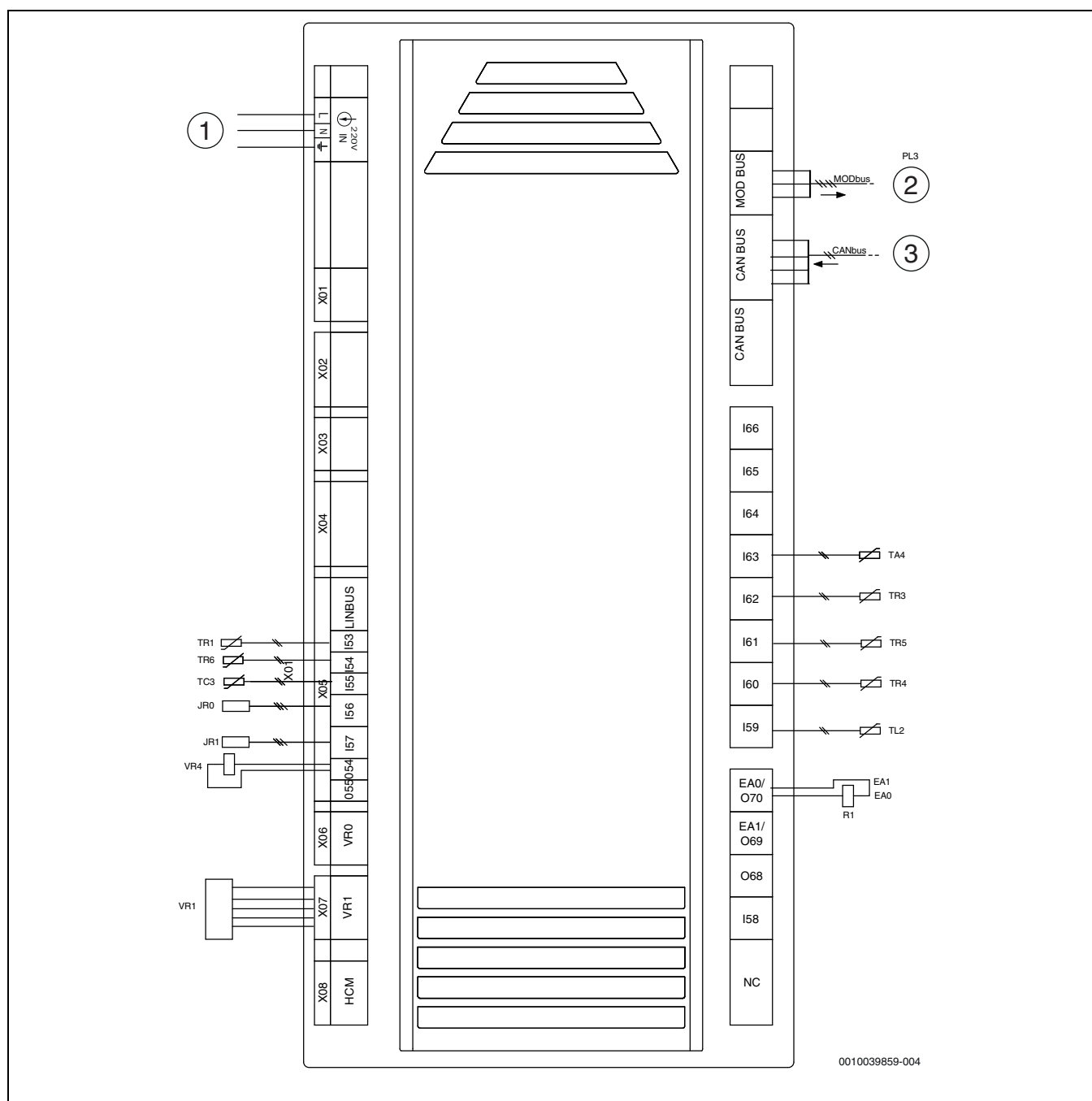
Obr. 46 Schéma zapojení XCU-SRH (XCU-HP)
