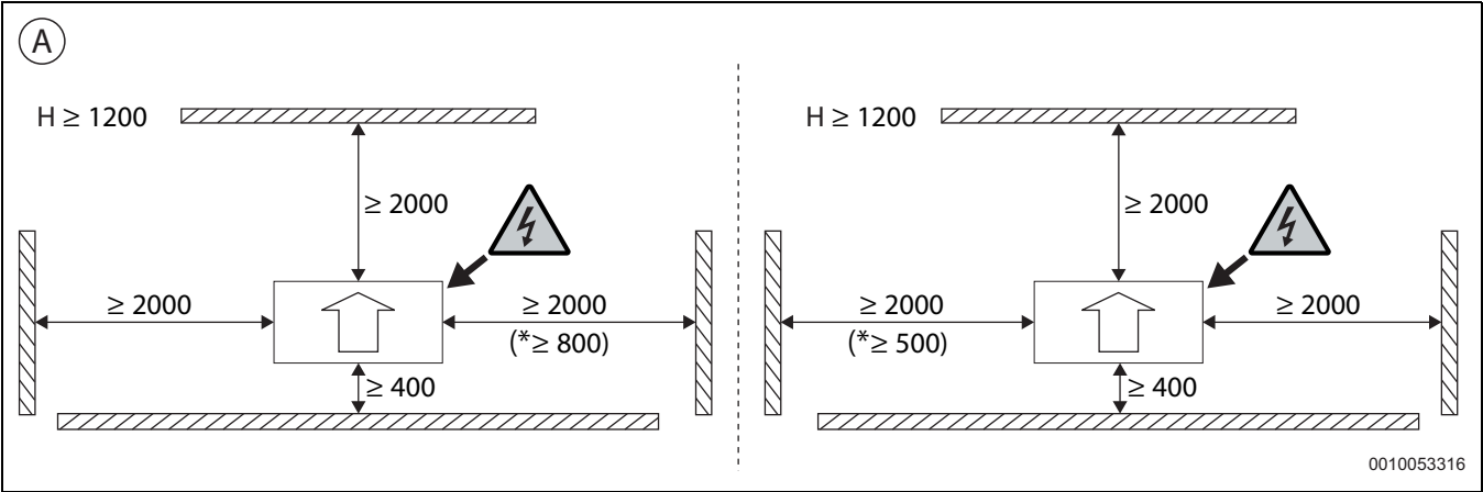
Obr. 16 Odstupy při instalaci
