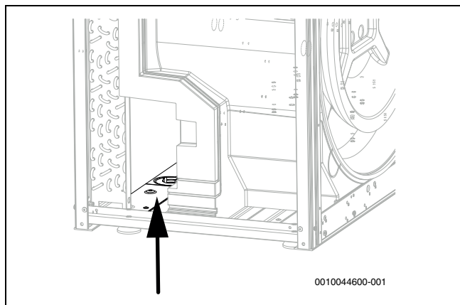
Obr. 41 Vyčistěte vanu
