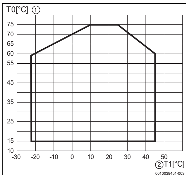
Obr. 42 Tepelné čerpadlo v provozu vytápění bez dohřevu
