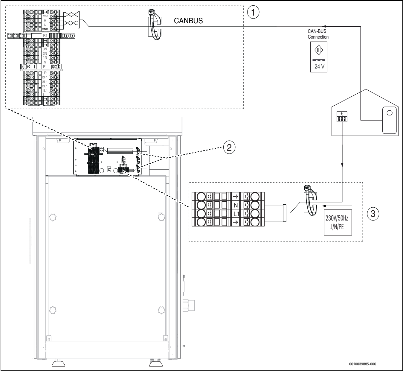
Obr. 36 Připojovací skříň
