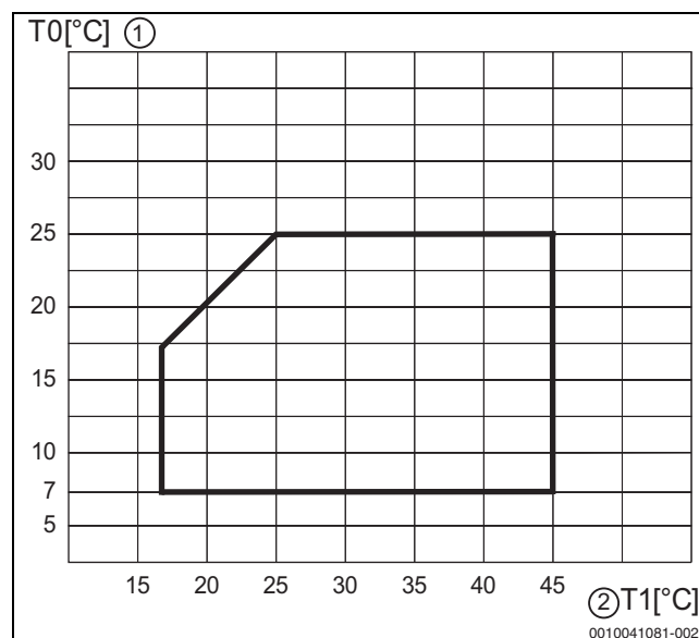
Obr. 43 Tepelné čerpadlo v provozu chlazení
