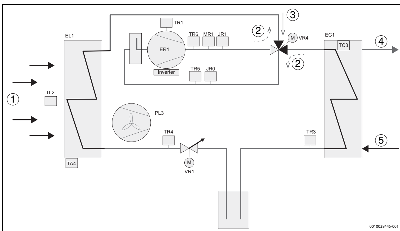
Obr. 44 Chladicí okruh
