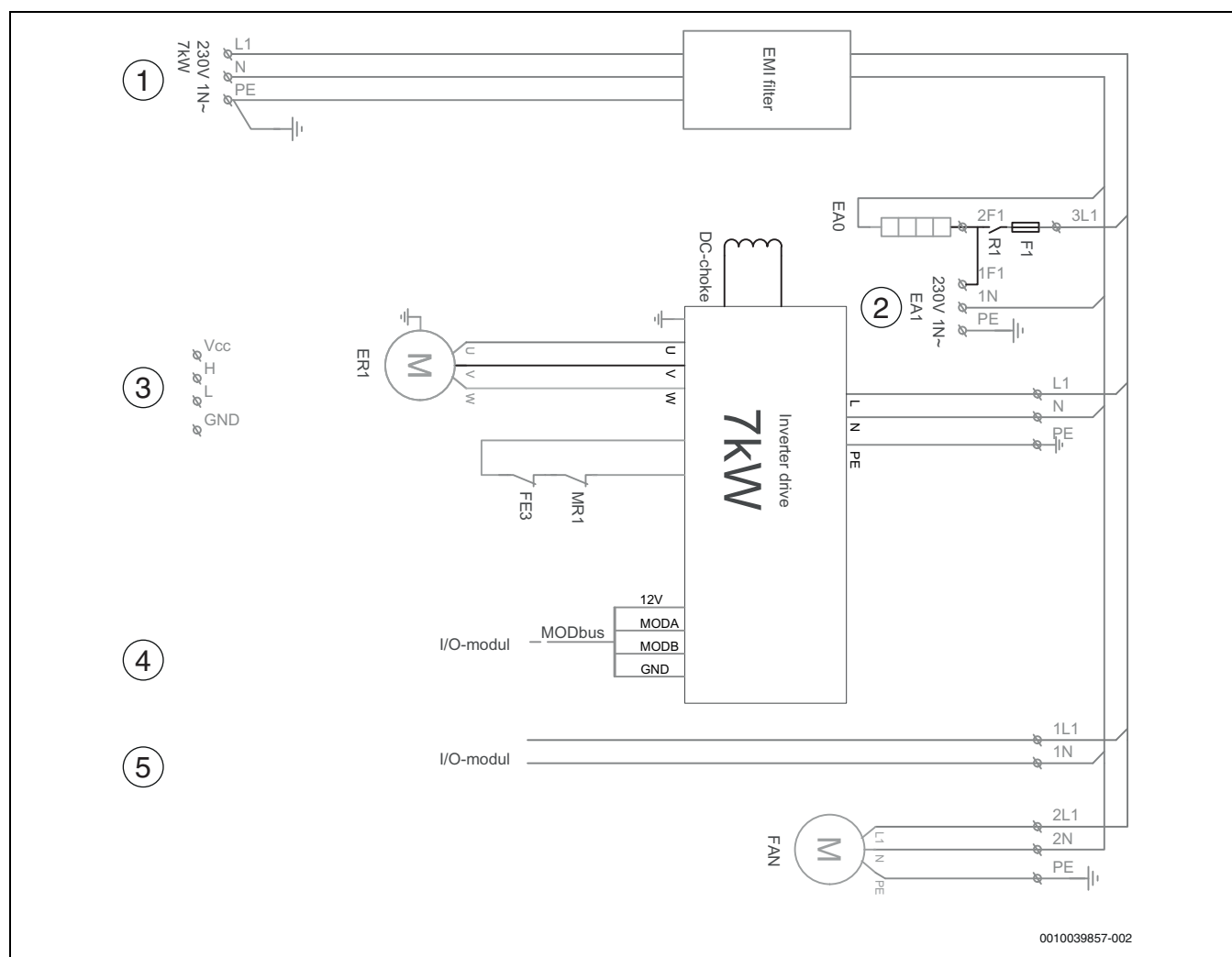
Obr. 45 Schéma zapojení invertoru
