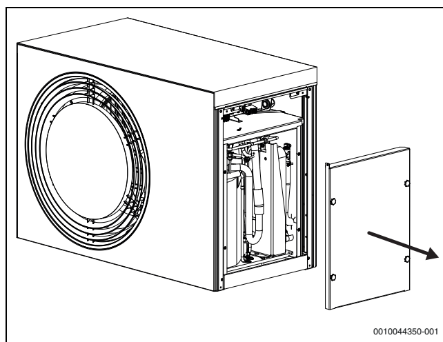
Obr. 31 Kryt skříně s chlazením
