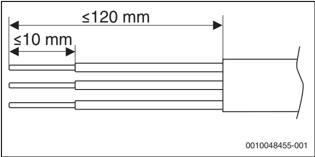
Obr. 37 Odizolování vodičů připojení síťového napájení
