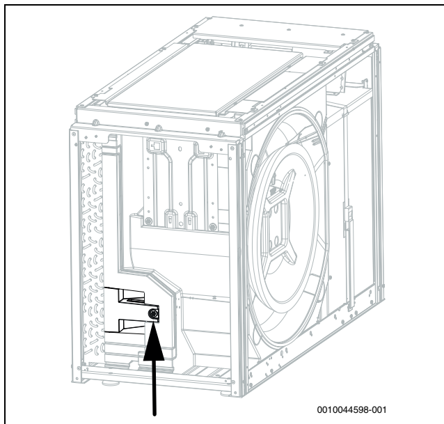
Obr. 39 Odšroubujte
