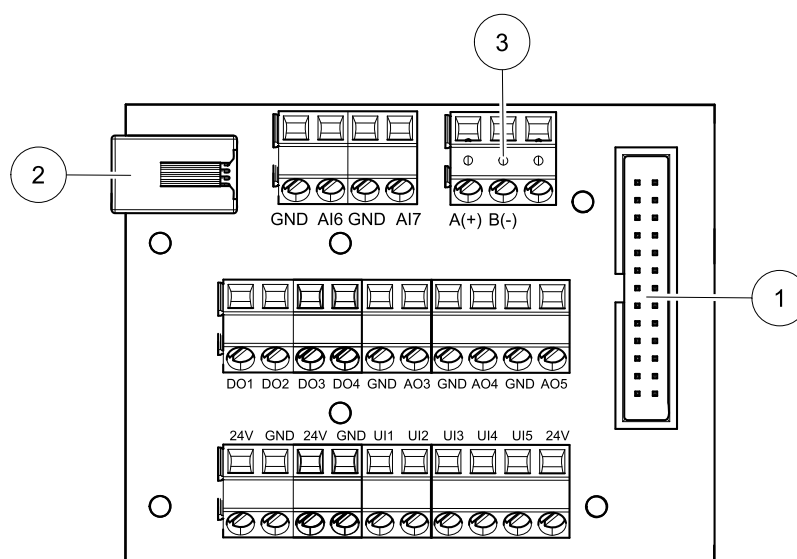
Obr. 8 Externí svorkovnice
