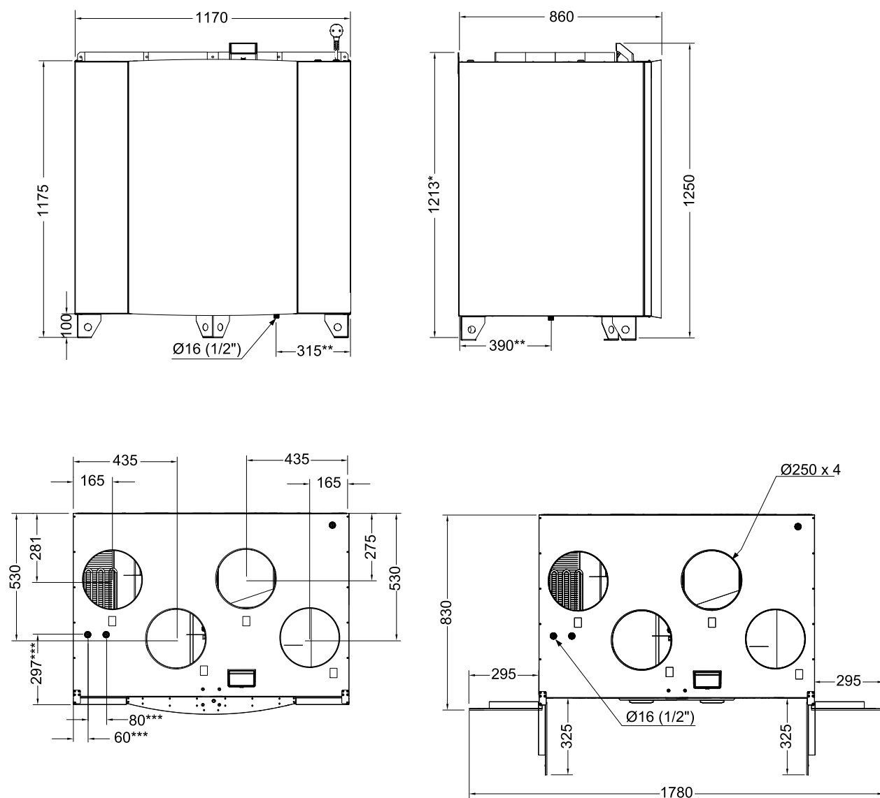
Obr. 2 Rozměry a hmotnost, model L (levý)
