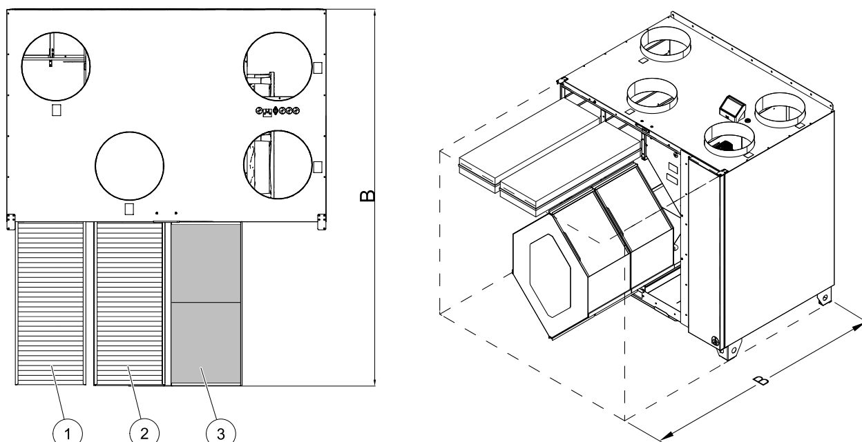
Obr. 4 Minimální prostor před jednotkou
