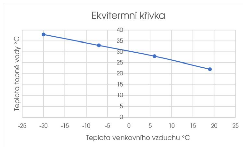
Obrázek 4.11: Graf - Ekvitermní křivka
