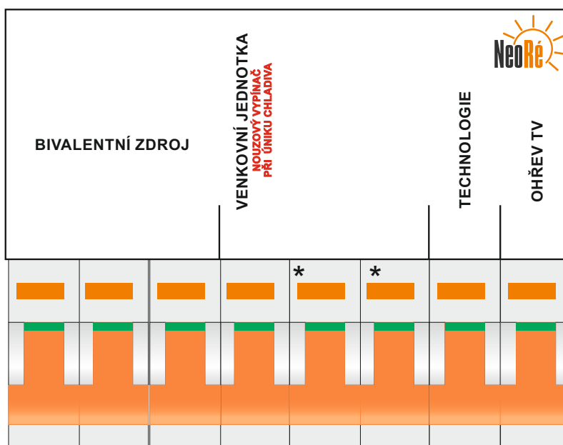
Jisticí prvky tepelného čerpadla -tři fázové provedení
